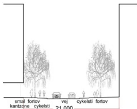
Snit D-D
