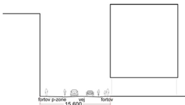
Snit C-C
